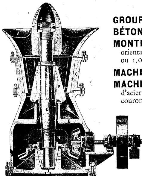
Coupe d'un concasseur giratoire.
